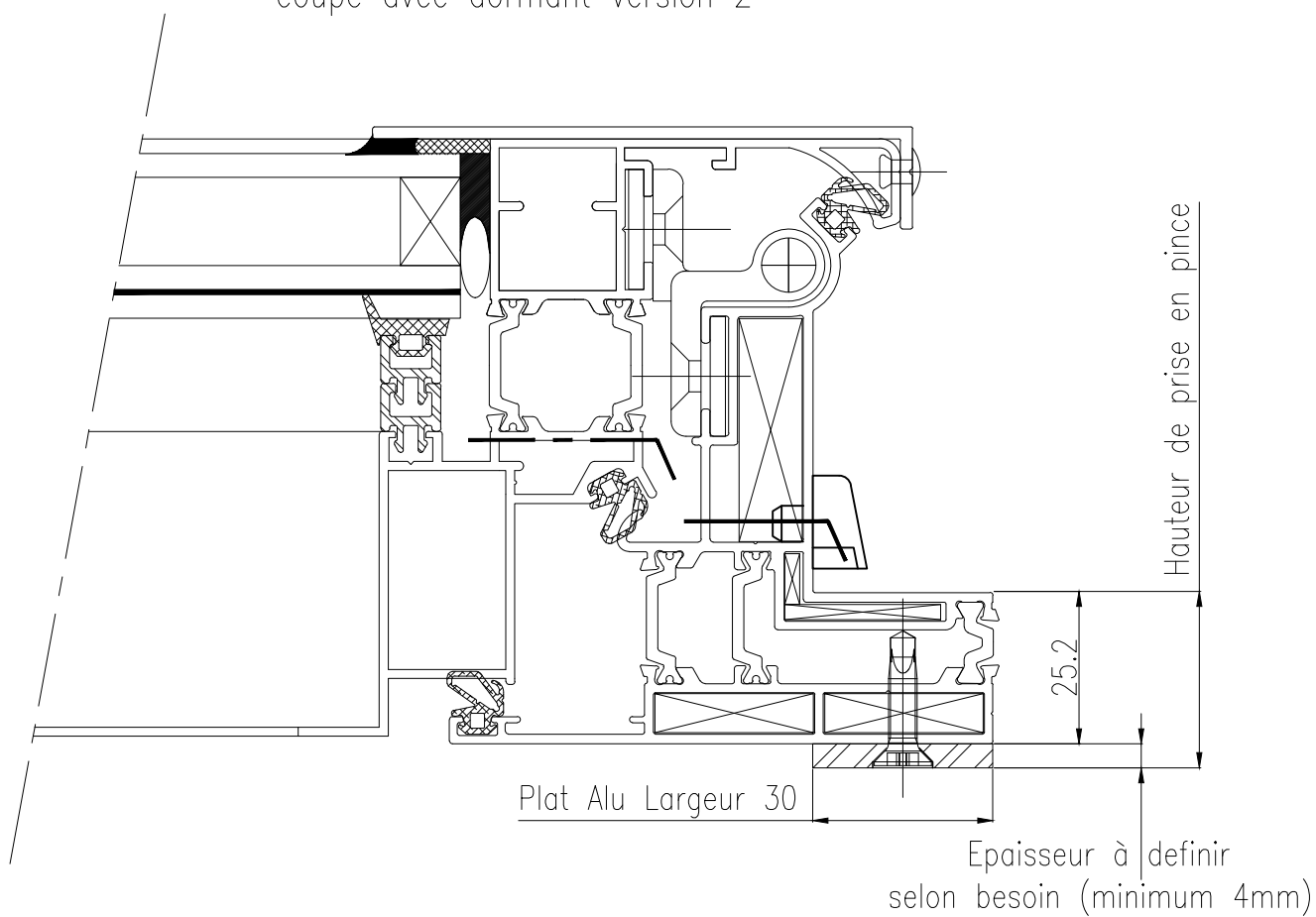
coupe avec dormant version 2
