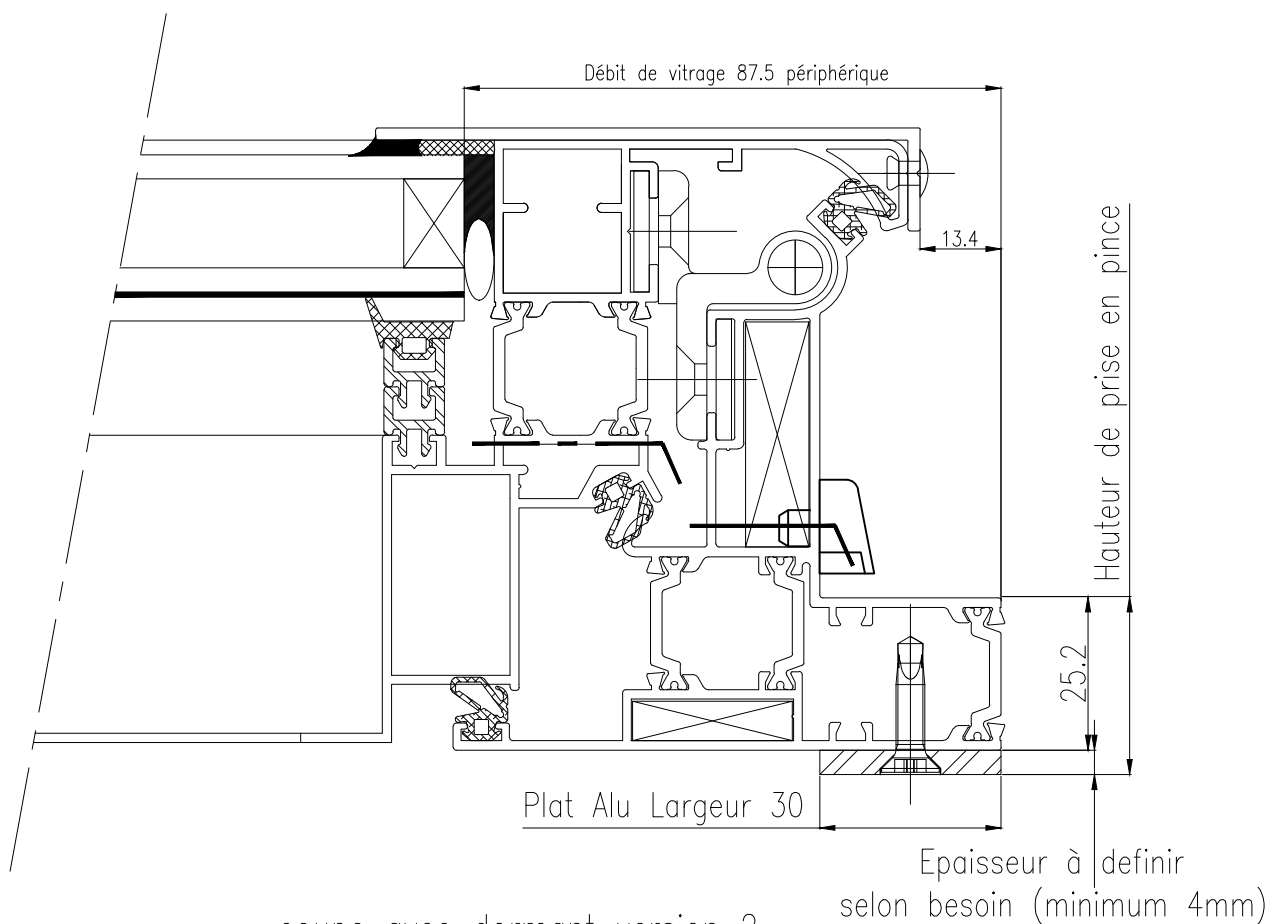
coupe avec dormant version 2
