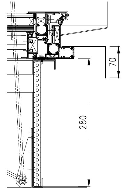
DETAIL COSTIERE
