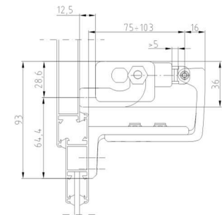
Installation sur dormant avec étrier réglable Z
