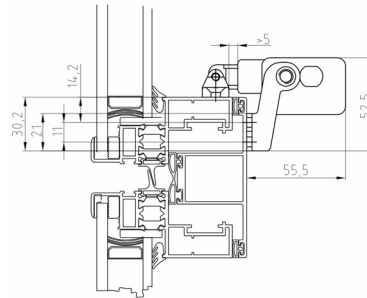
Volet caché avec étriers court et minces
