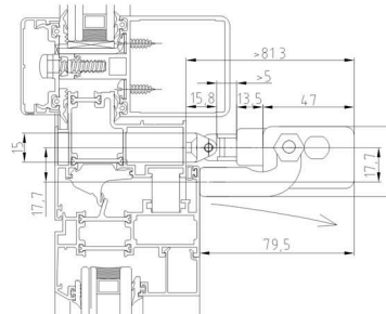
Installation sur volet avec étriers longs
