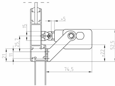
Installation frontale avec étriers longs et minces
