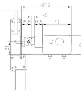
Installation avec étriers longs
