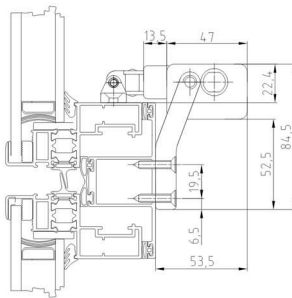
Installation sur dormant
