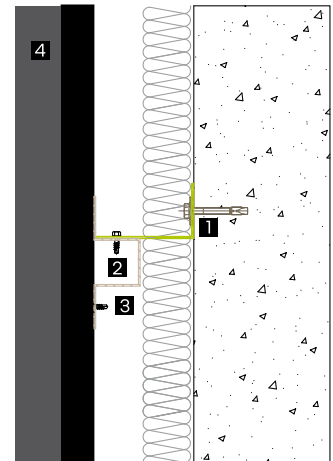
COUPE VERTICALE
