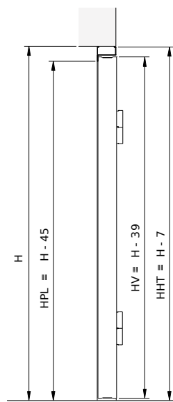
Coupe verticale
