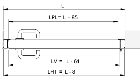
Coupe horizontale
