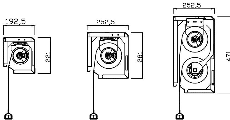
Monocylindre Ø 89 Monocylindre Ø 100 Multicylindres superposés Ø 100
