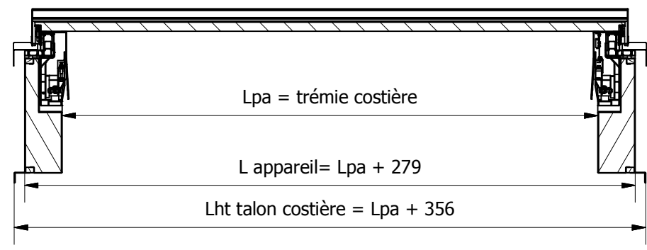
D-D
