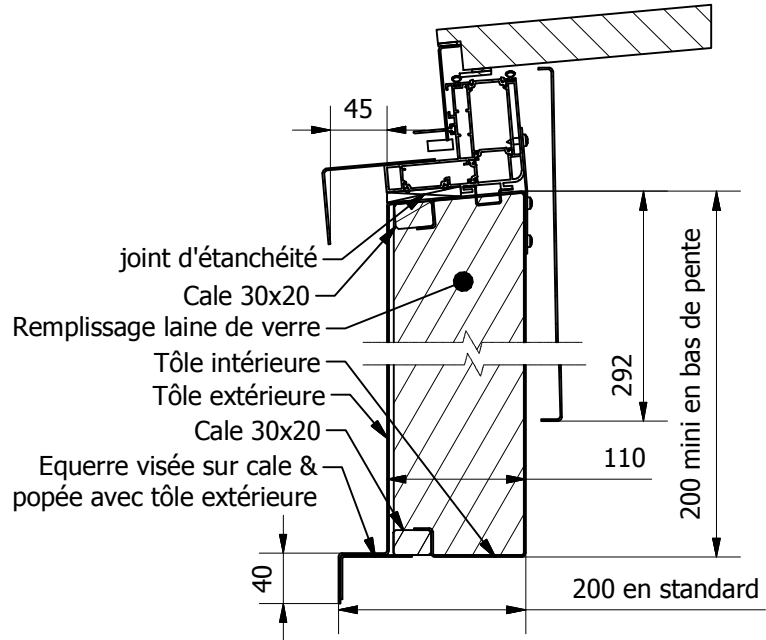
A-A ( 1/6 )
