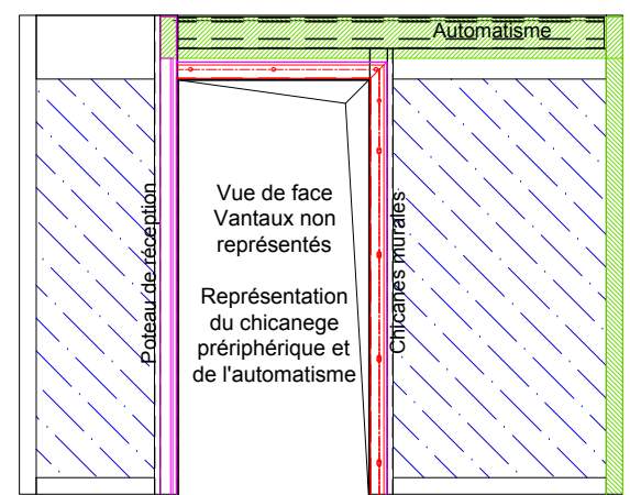
Vue coté automatisme Fermeture à Gauche
