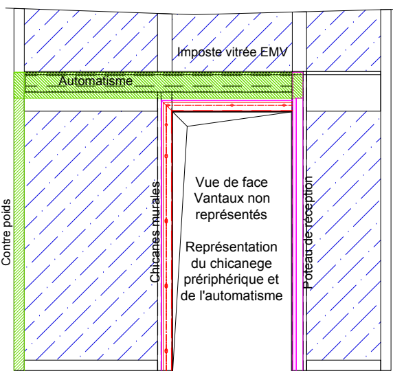
Vue coté automatisme Fermeture à Droite
