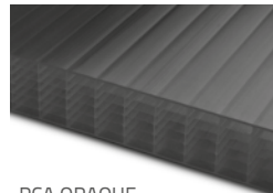
PCA OPAQUE
