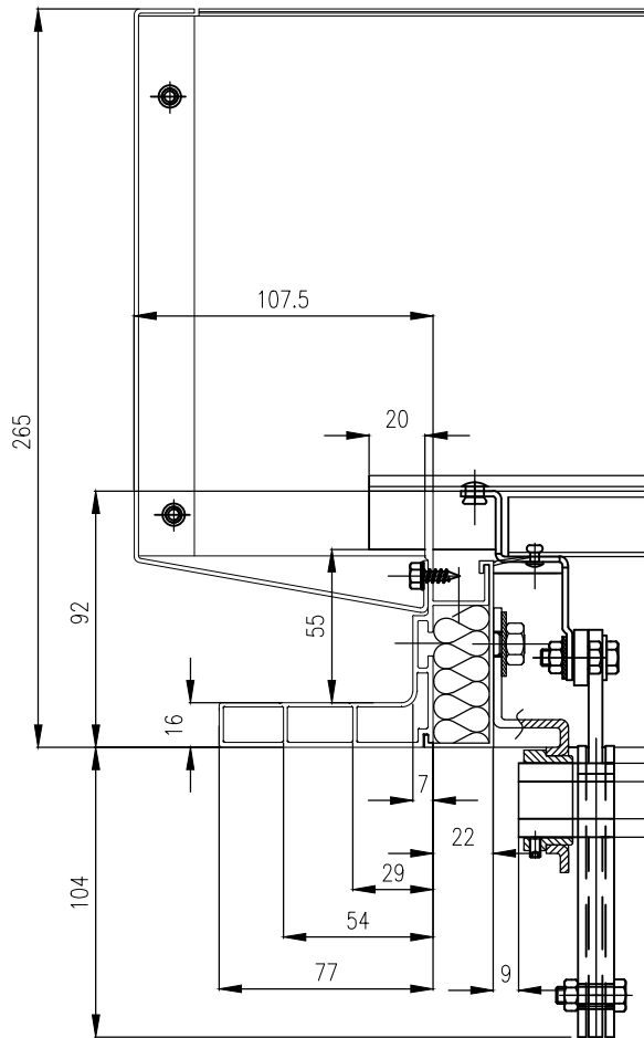
Cadre F ECHELLE 1:3
