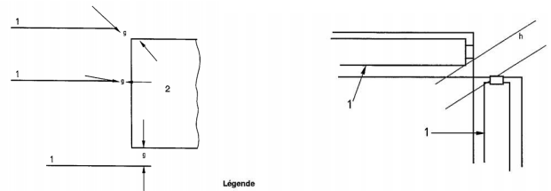
Légende g Espace libre 1 Ecran de cantonnement de fumée 2 Plac
