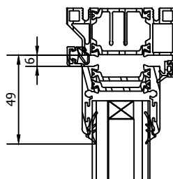
B-B ( 1/2 )
