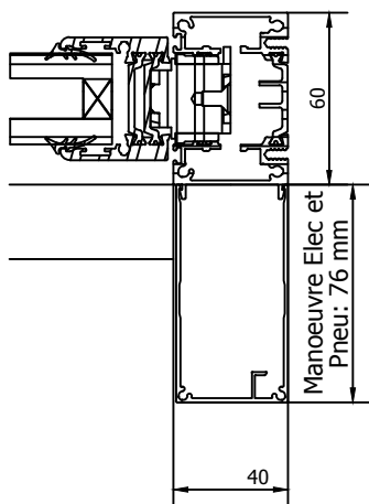
C-C ( 1/2 )
