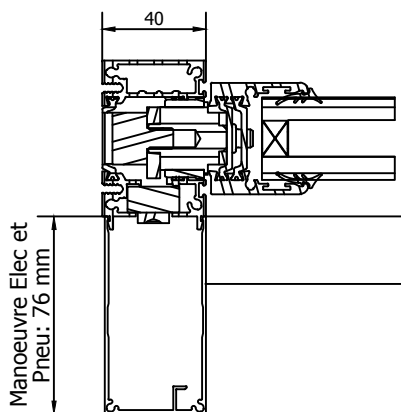
D-D ( 1/2 ) Capot pour manoeuvre
