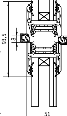
C-C ( 1/2 )
