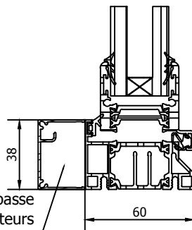
C-C ( 1/2 )
