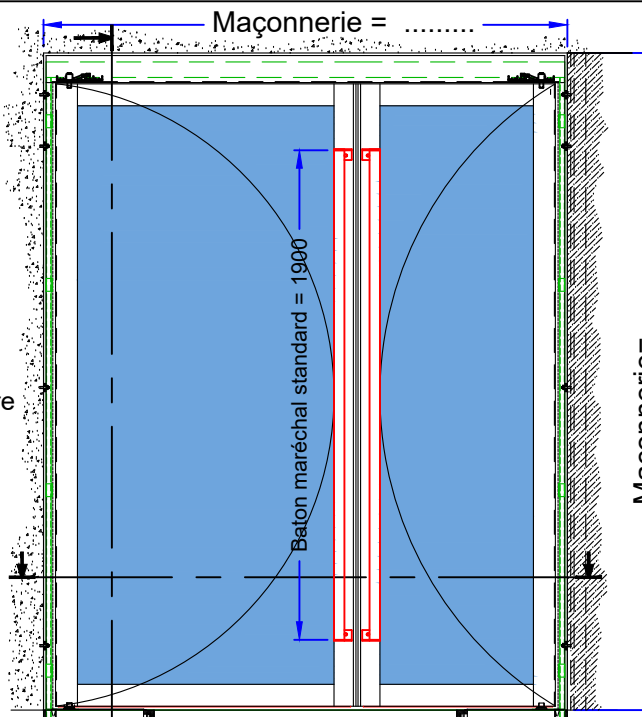
VANTAUX INÉGAUX
