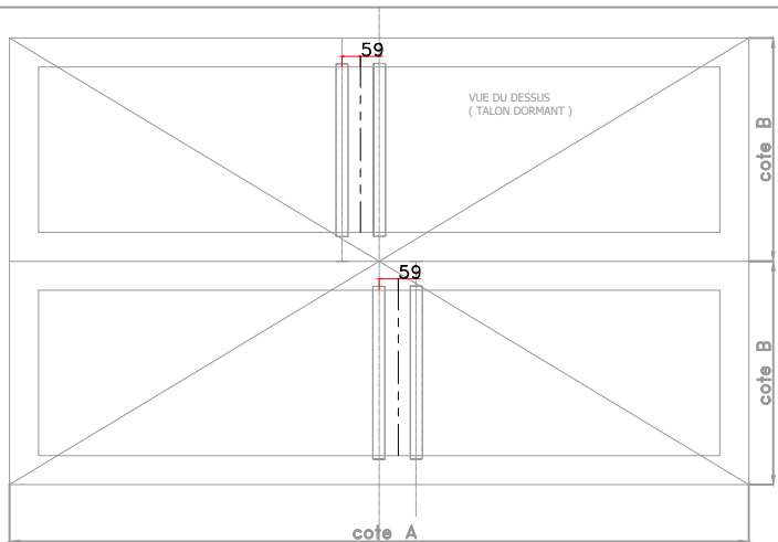
Implantation pour vantail à 1 vérin
