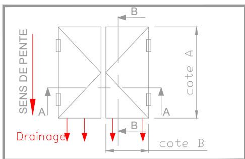
Implantation pour vantail à 2 vérens
