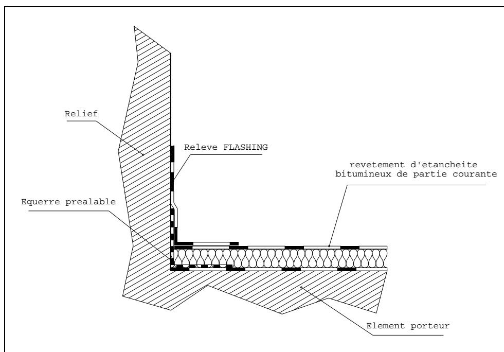
Figure 1 – Procédé FLASHING Principe - Cas particulier avec isolant de partie courante et sans dispositif écartant les eaux de ruissellement (cf. § 7.321)
