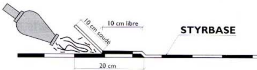
Figure 4A – Recouvrements transversaux avec écran thermique
