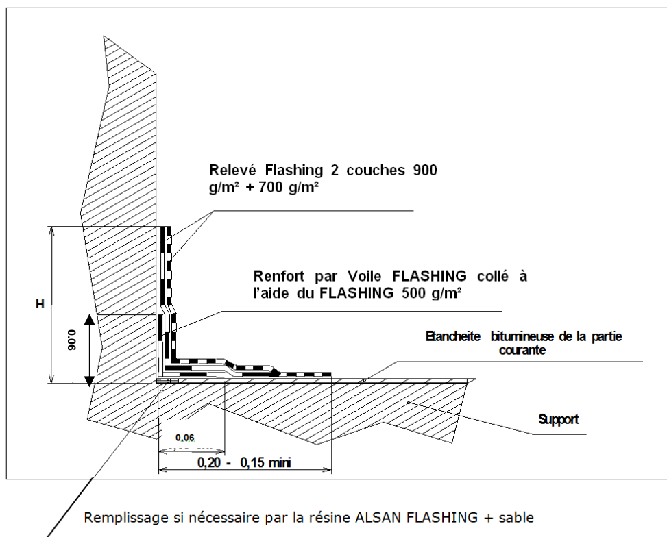
Figure 2 – Mise en œuvre du procédé FLASHING (cf. § 7.321) Cas particulier sans isolant de partie courante et sans dispositif écartant les eaux de ruissellement
