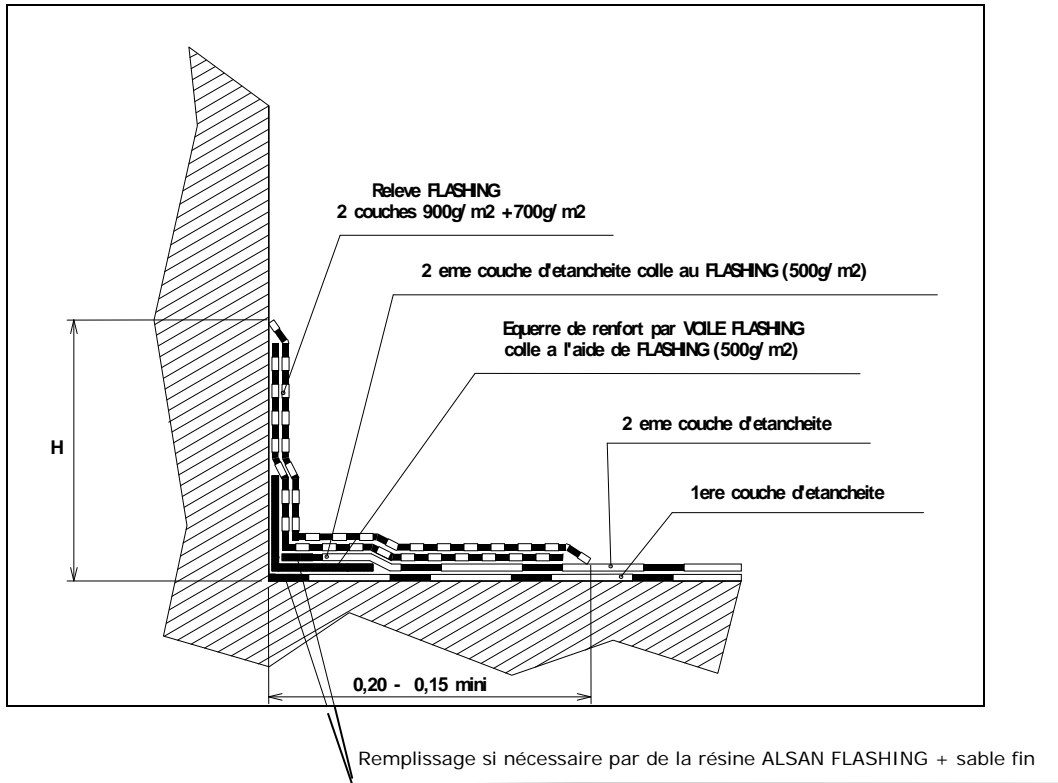
Figure 3 – Procédé FLASHING - variante de pose de l'équerre de renfort insérée entre les deux feuilles du revêtement bicouche, Cas particulier sans isolant de partie courante et sans dispositif écartant les eaux de ruissellement (cf. § 7.321)
