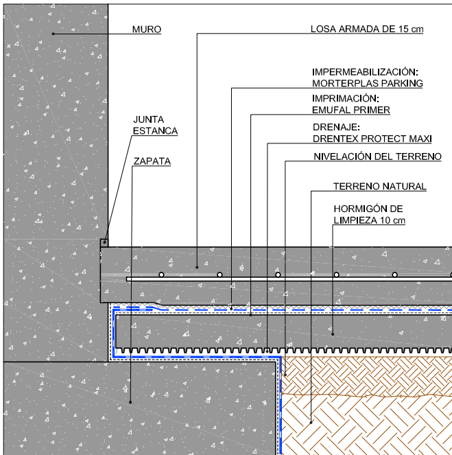
ENCUENTRO DE LA LOSA CON MURO Y ZAPATA
