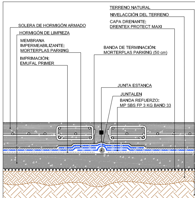
JUNTA DE DILATACIÓN
