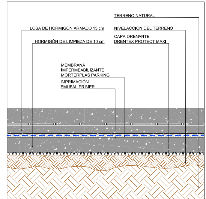
SECCIÓN TIPO
