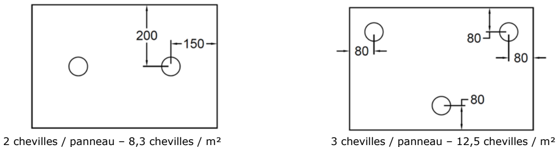
Figure 1b : Plans de chevillage - panneaux PAVAWALL-SMART de dimensions 400 x 800 mm
