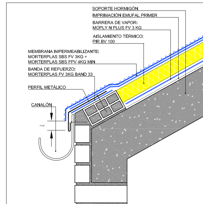
DETALLE VOLADIZO
