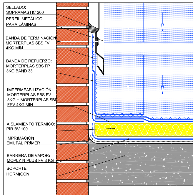
DETALLE ENTREGA A PARAMENTO VERTICAL
