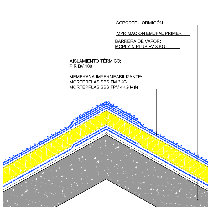
DETALLE CUMBRERA
