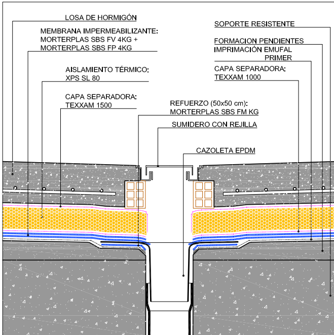
DETALLE DESAGÜE
