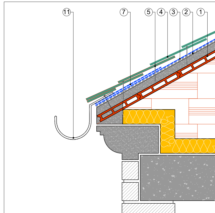
DETALLE VOLADIZO
