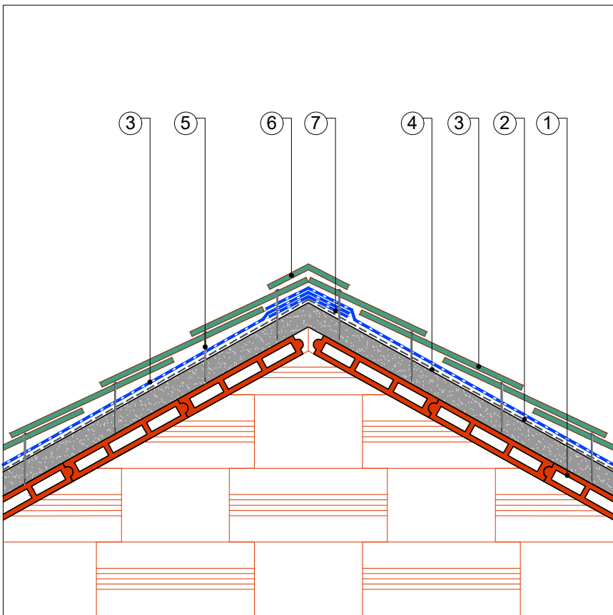
DETALLE CUMBRERA
