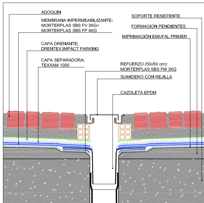
DETALLE DESAGÜE
