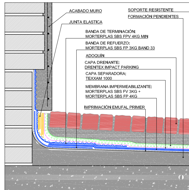
DETALLE PERIMETRAL
