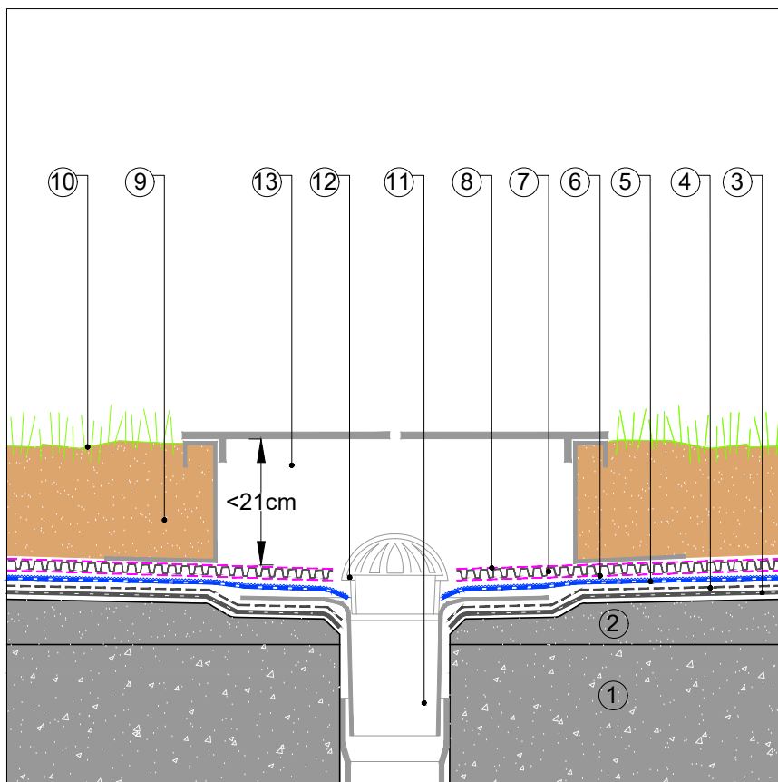
DETALLE DESAGÜE
