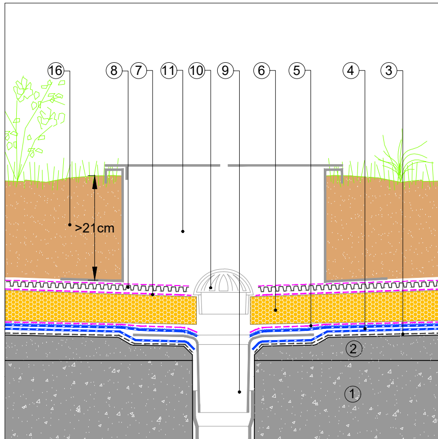
DETALLE DESAGÜE
