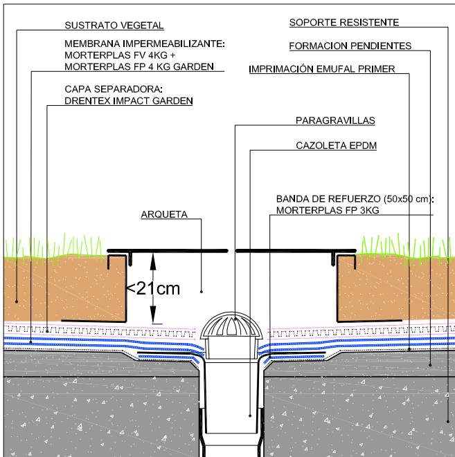
DETALLE DESAGÜE
