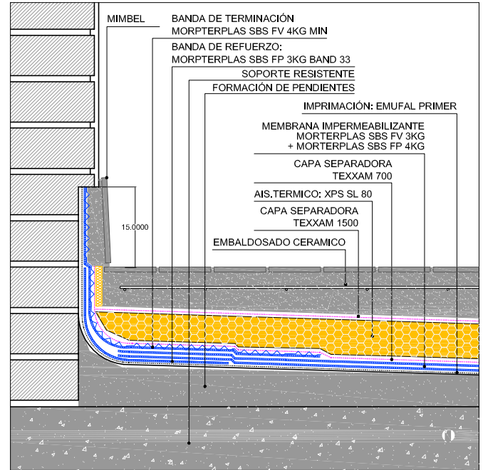
DETALLE PERIMETRAL
