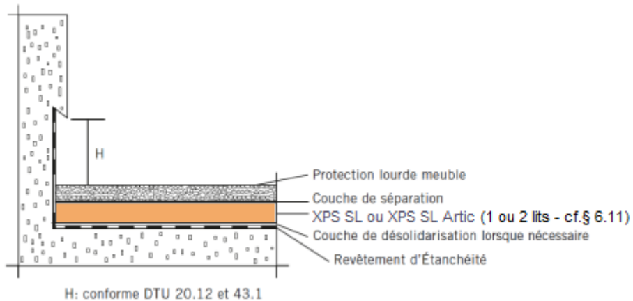
Figure 2 – Relevé sur toiture-terrace inaccessible avec retrait formant larmier
