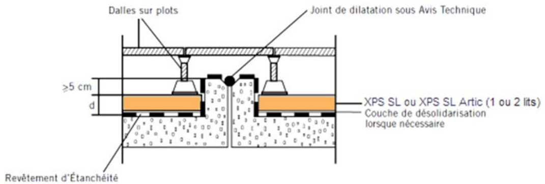
Figure 9 – Coupe de principe sur joint de dilatation
