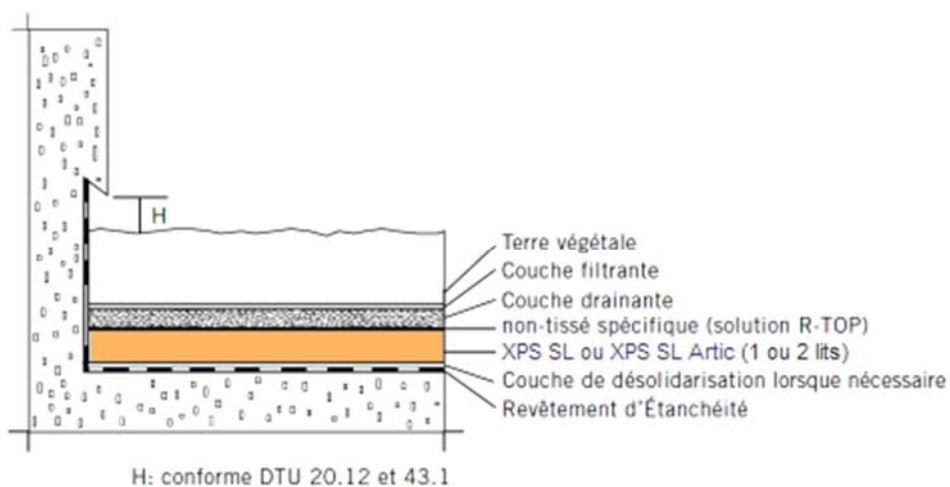
Figure 16 - Coupe de principe d'une toiture terrasse jardin
