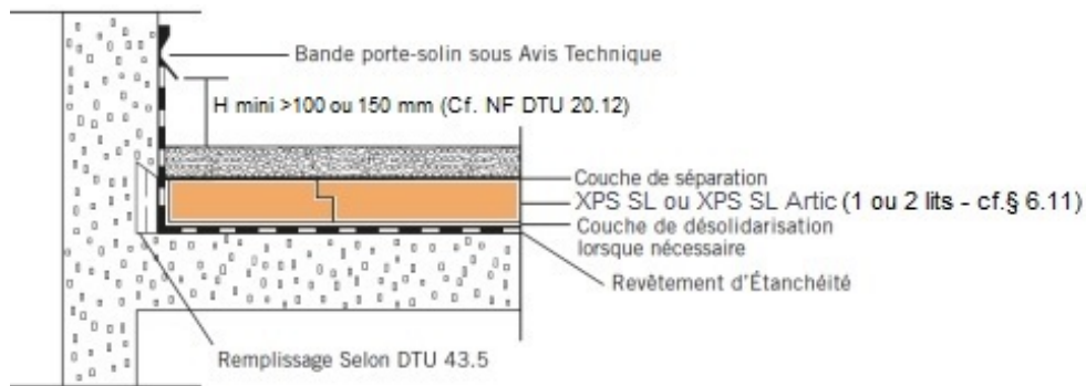
Figure 5 – Coupe sur relevé en travaux de réfections
