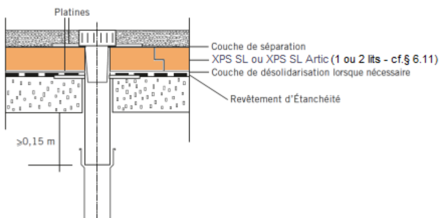
Figure 7 – Exemple d'EEP (hors établissements recevant du public)
