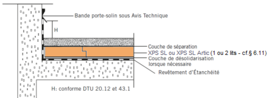
Figure 3 – Coupe de principe sur relevé avec bande porte-solin métallique
