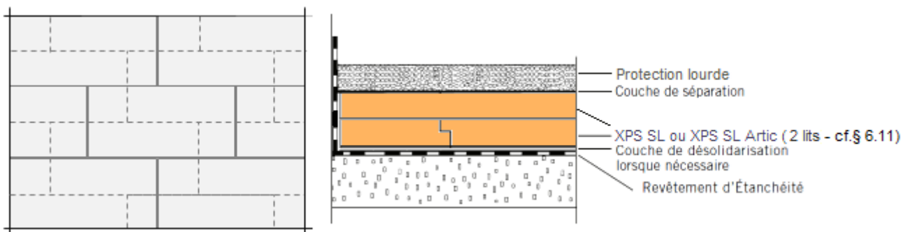
Figure 13 – Principe de mise en œuvre en 2 lits (à joints décalés)
