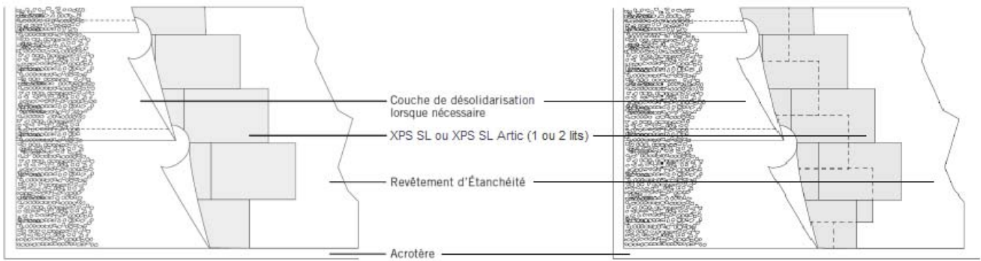
Figure 11 – Vue de dessus de principe d'une toiture inversée
