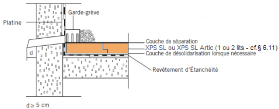
Figure 8 – Coupe sur relevé avec Trop-Plein d'Eau pluviale (TPE)
