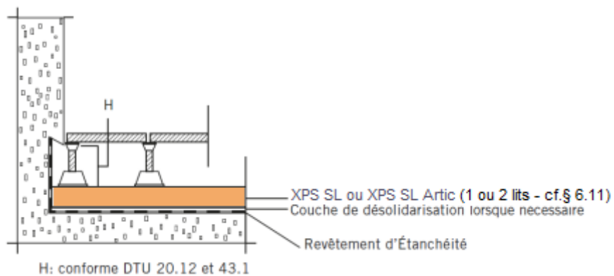
Figure 4 – Relevé sur terrasse accessible aux piétons et au séjour avec dalles sur plots
