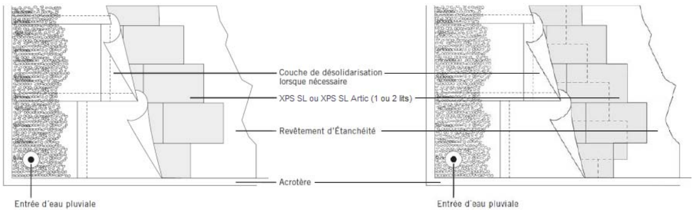
Figure 12 – Vue de dessus de principe de la Solution R-TOP en pente nulle
