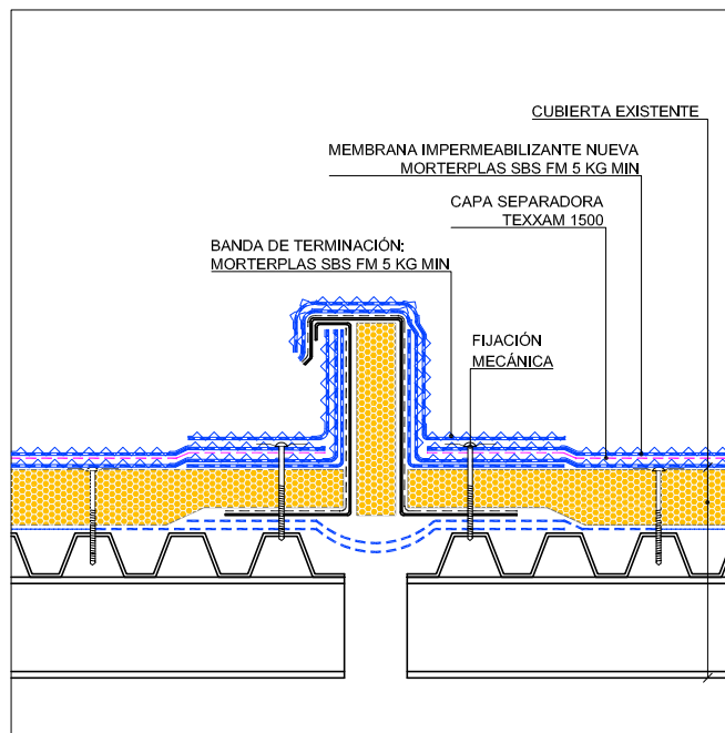
DETALLE JUNTA ESTRUCTURAL
