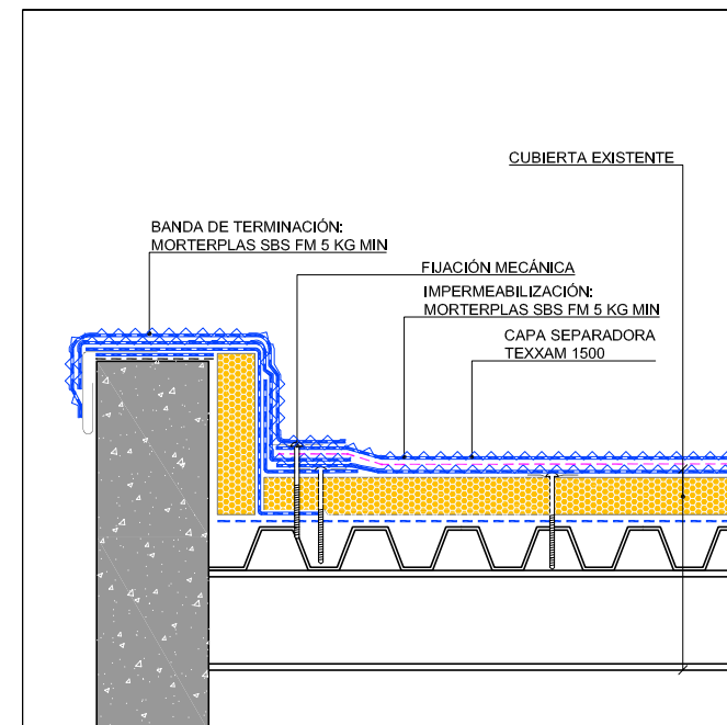
DETALLE ENTREGA A PERIMETRO
