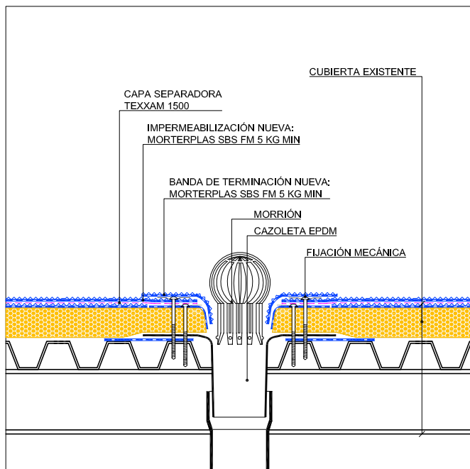
DETALLE DESAGÜE
