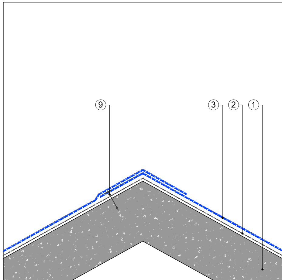
DETALLE CUMBRERA
