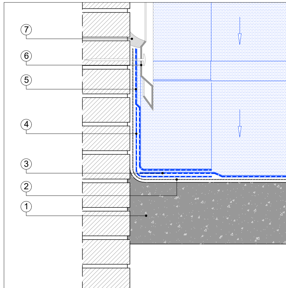
DETALLE ENTREGA A PARAMENTO VERTICAL
