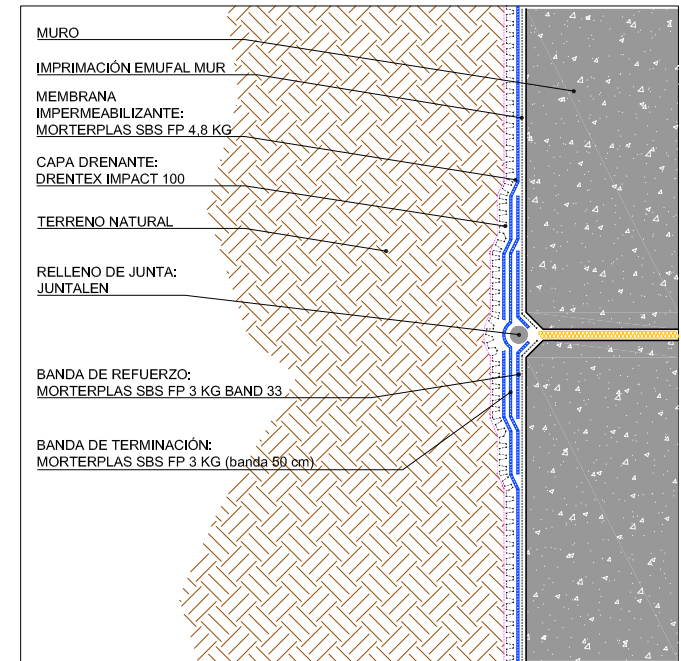
DETALLE JUNTA DE DILATACIÓN
