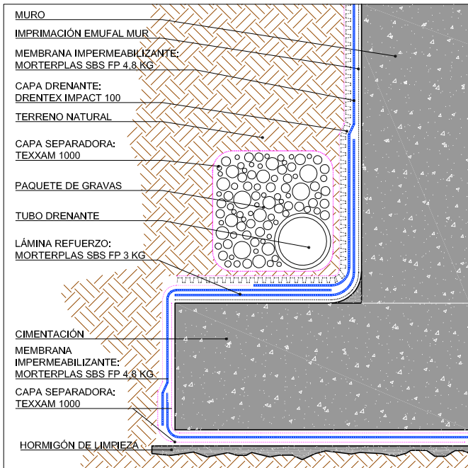
DETALLE ENCUENTRO CIMENTACIÓN
