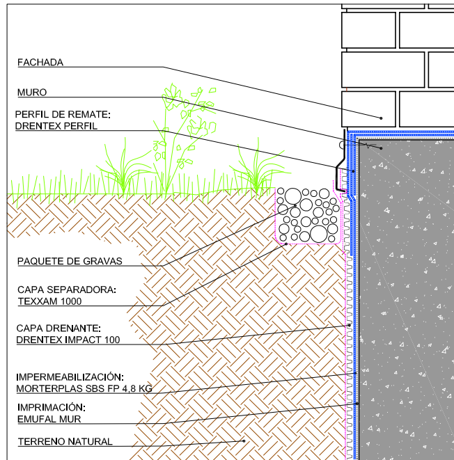
DETALLE ENCUENTRO FACHADA
