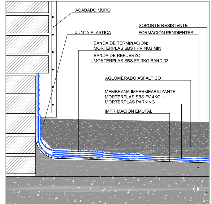
DETALLE PERIMETRAL
