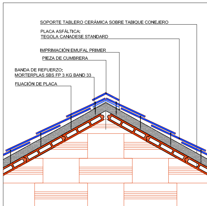
DETALLE CUMBRERA
