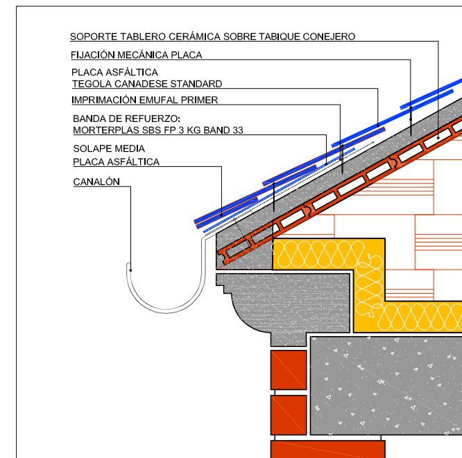
DETALLE VOLADIZO
