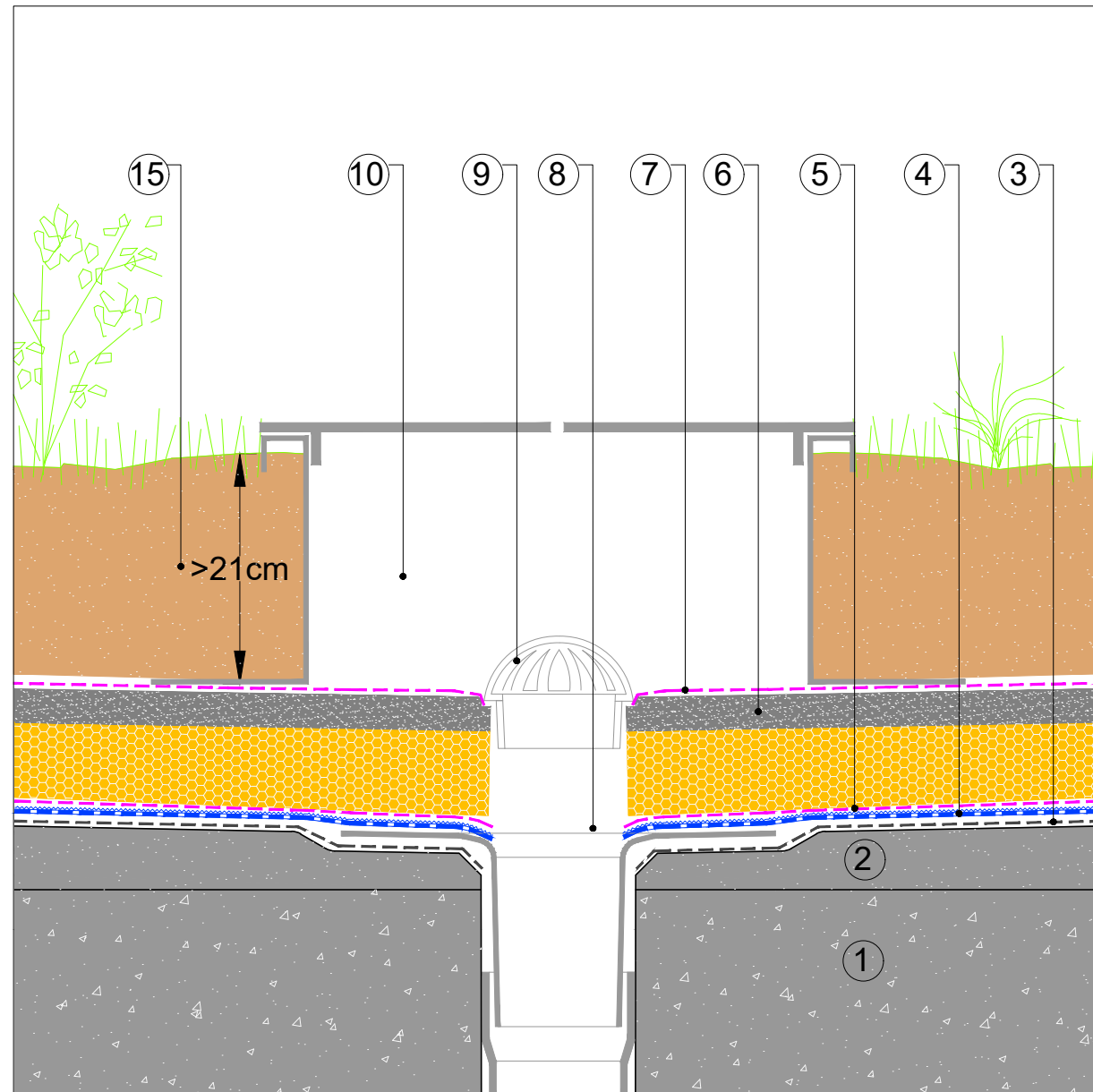
DETALLE DESAGÜE
