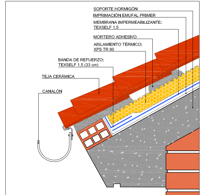
DETALLE VOLADIZO
