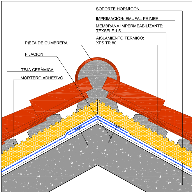
DETALLE CUMBRERA
