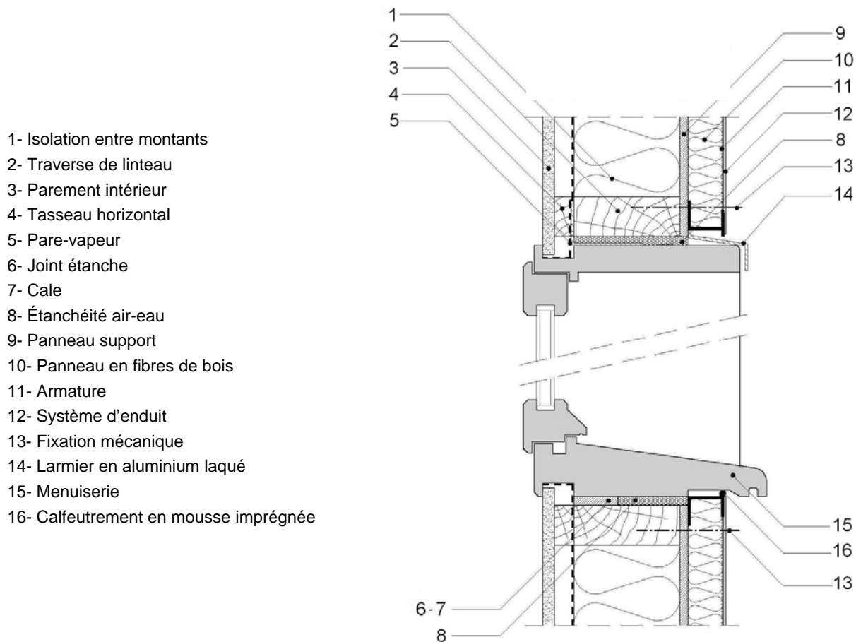
Figure 5b : Fixations mécaniques au niveau des baies (coupe horizontale)
