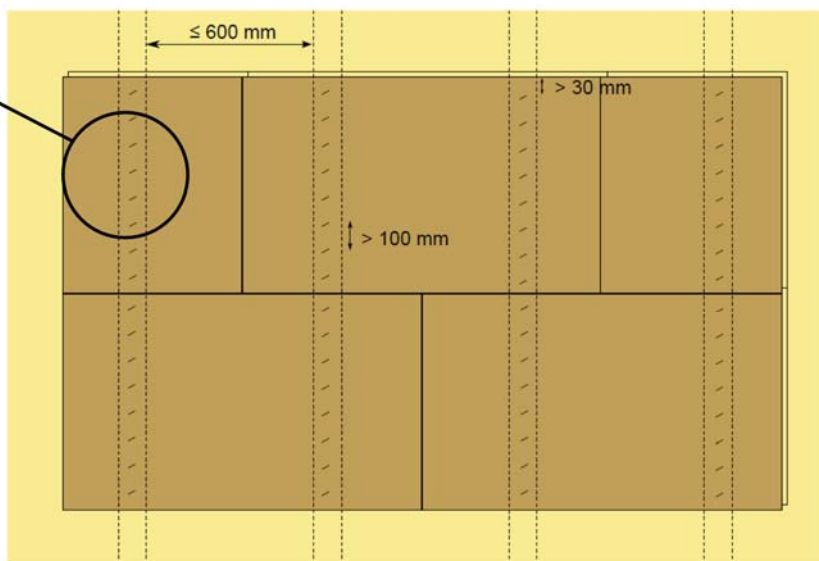
16 agrafes par panneau (8 agrafes par montant)
