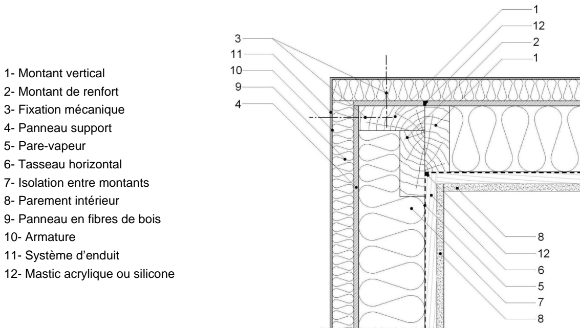
Figure 4a : Fixations mécaniques aux angles sortants (coupe horizontale)
