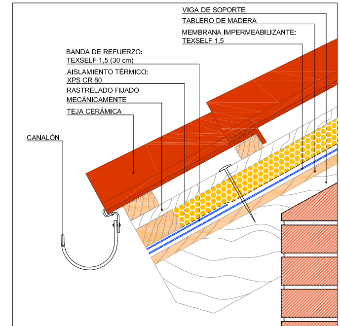
DETALLE VOLADIZO
