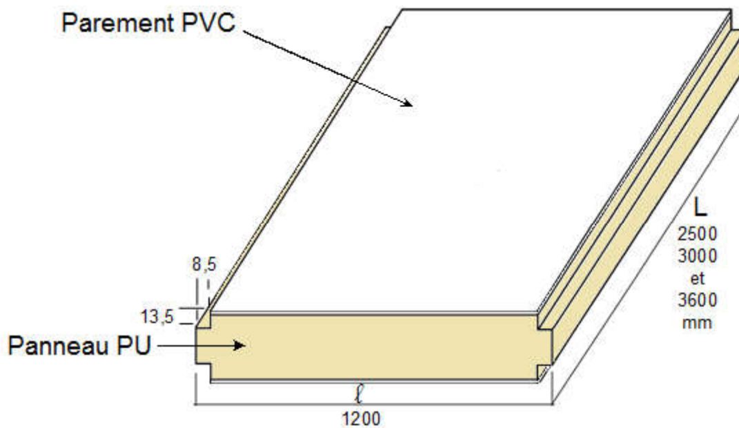
Figure 3 - EFICHO PLAFOND (en mm)
