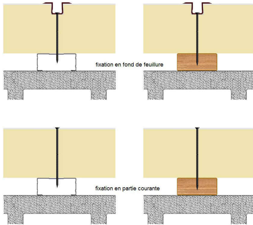
Figure 12 - Fixation des panneaux EFICHOCE PLAFOND et EFICHOCE PAROI dans l'ossature
