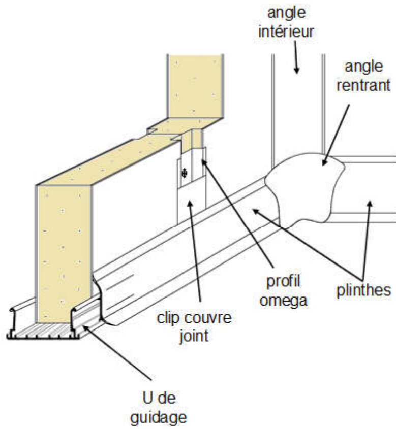
Figure 20 - Dispositif pour le sol / le plafond pour EFICHOC CLOISON
