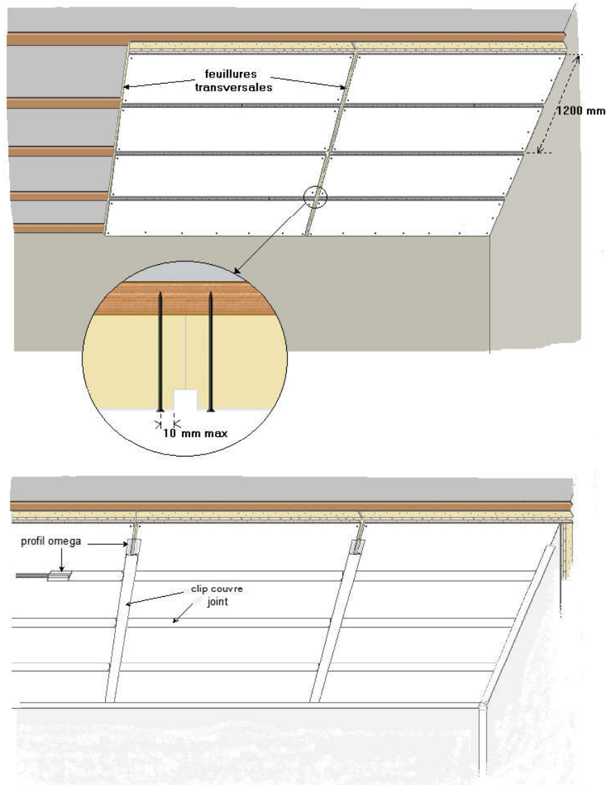
Figure 19 - Aboutage des panneaux EFICHOC PLAFOND
