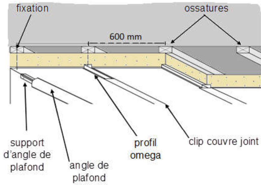
Figure 18 - Prescriptions de pose EFICHOC PLAFOND
