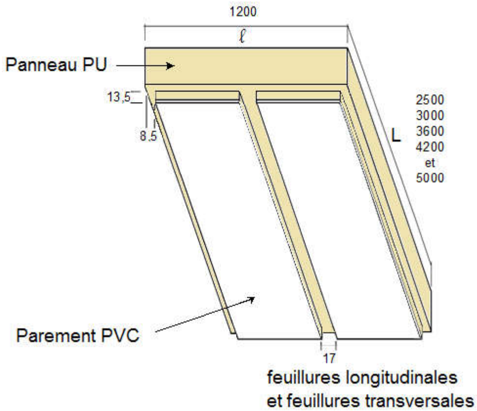
Figure 2 - EFICHO CLOISON (en mm)
