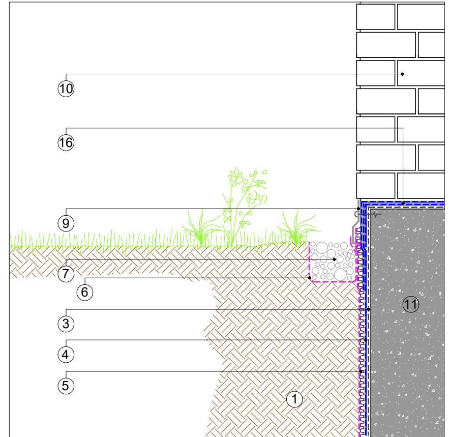
DETALLE ENCUENTRO FACHADA
