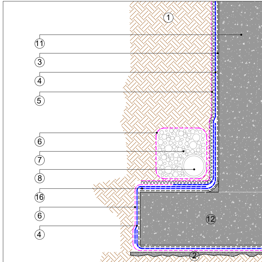
DETALLE ENCUENTRO CIMENTACIÓN
