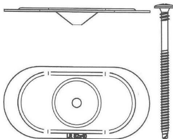
Fig. 1: ETANCO EVB DF 2C en 82x40 R plaatje
