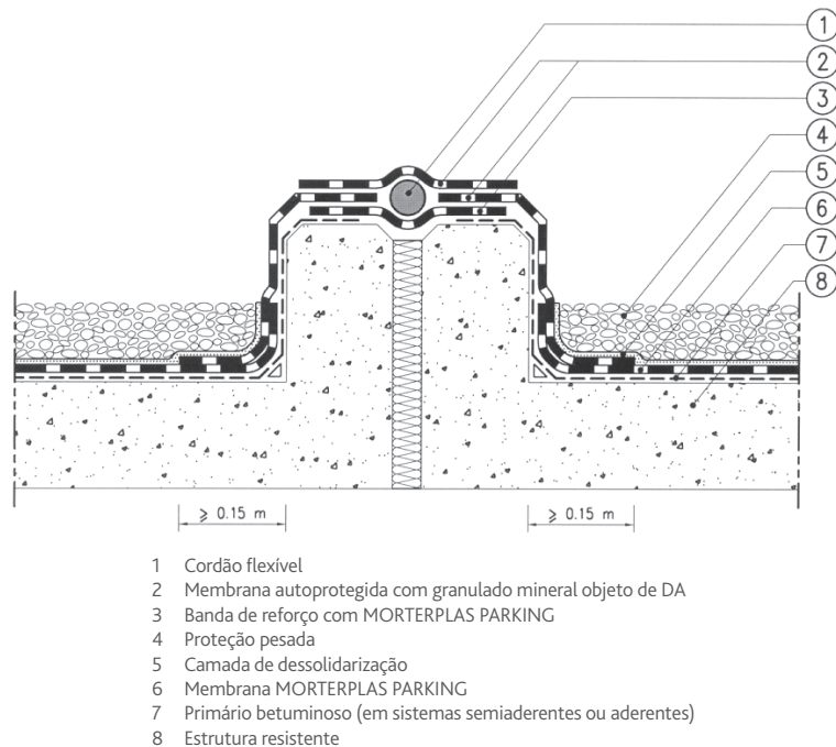
Figura 2 – Junta de dilatação sobre-elevada
