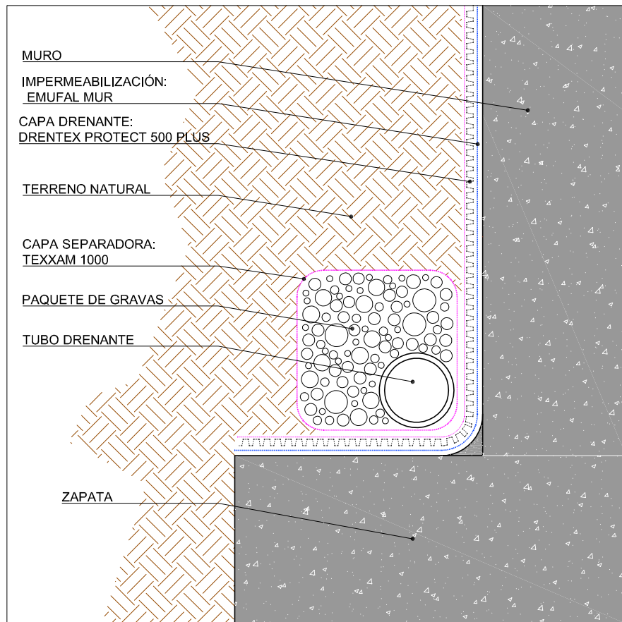
DETALLE ENCUESTRO CIMENTACIÓN
