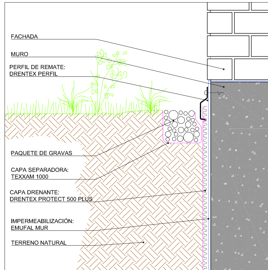
DETALLE ENCUESTRO FACHADA
