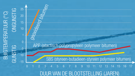
Fig. 40 Ontwikkeling over een periode van 17 jaar (18 zomers) van het gedrag van bitumineus materiaal (APP en SBS bitumen polymeren) als dakbedekking.
